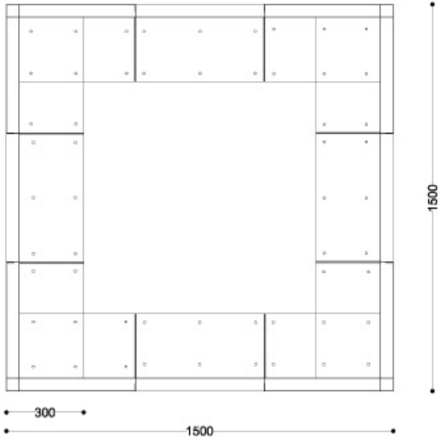
Draufsicht
