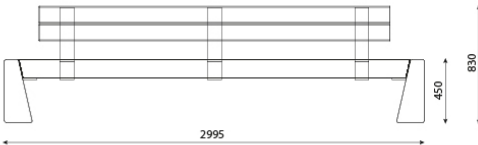
Rzut z frontu
