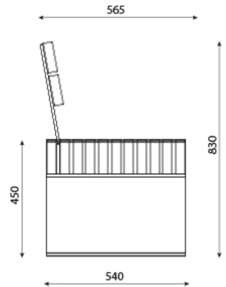
Rzut z boku
